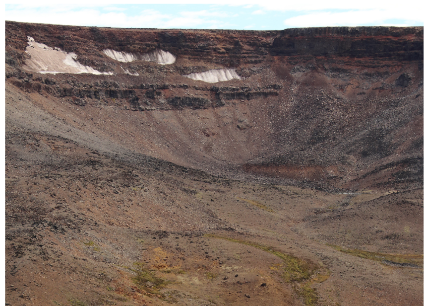
Glaciar de escombros y manchones de nieve en las nacientes del arroyo Italiano (Foto: Mariano Castro)
