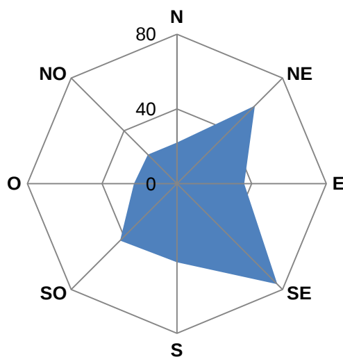
Figura 13: Orientación de los glaciares.
