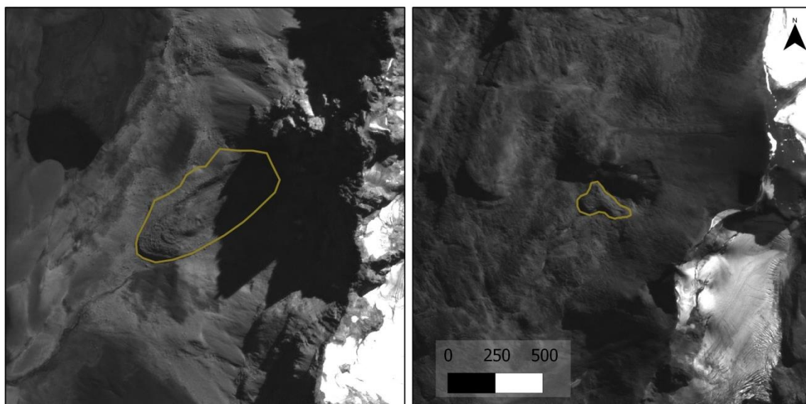
Figura 11: Pequeños glaciares de escombros en el Cordón Moyano. Los frentes se encuentran a 1.130 y 1.500 msnm (imagen ALOS PRISM 29/03/2008).
