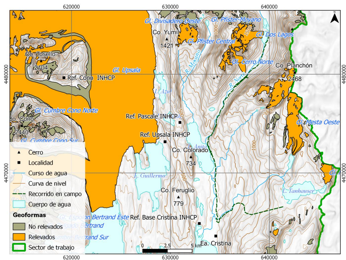
Figura 16: Mapa de las geoformas relevadas en el campo
