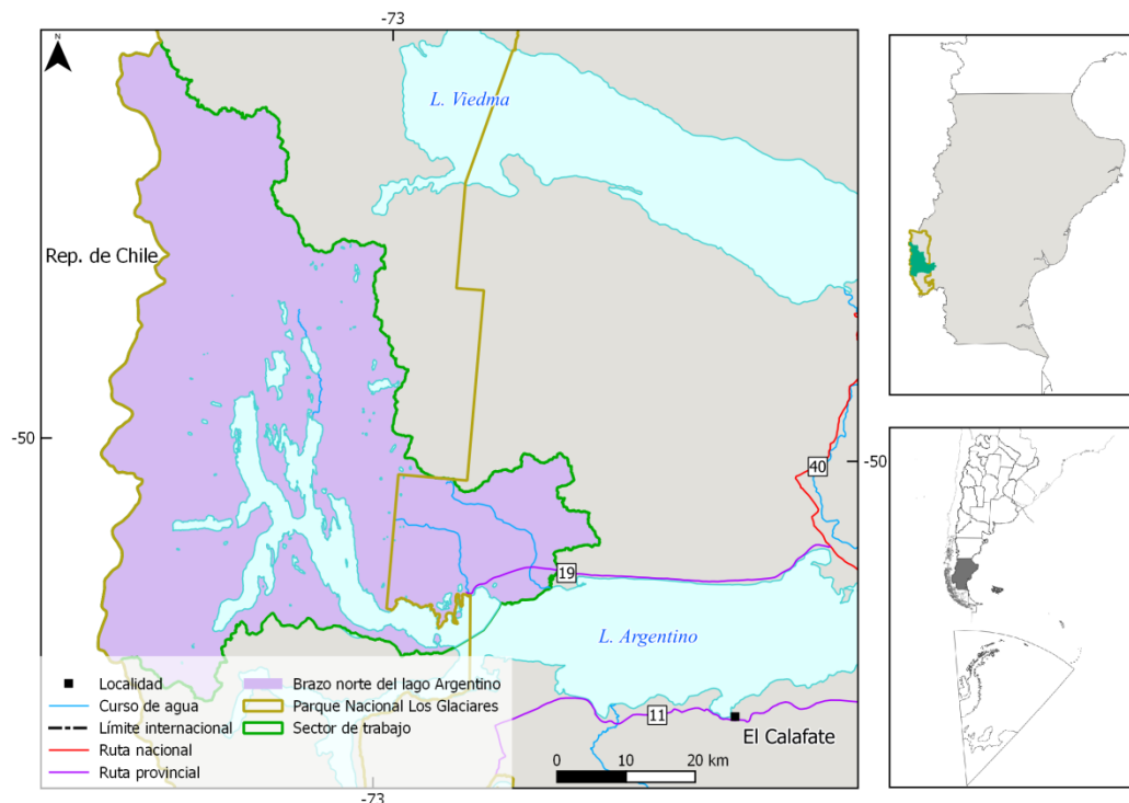
Figura 4: Mapa de ubicación de la subcuenca Brazo Norte del Lago Argentino.
