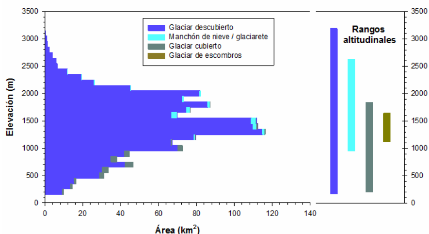
Figura 14: Hipsometría de los glaciares.
