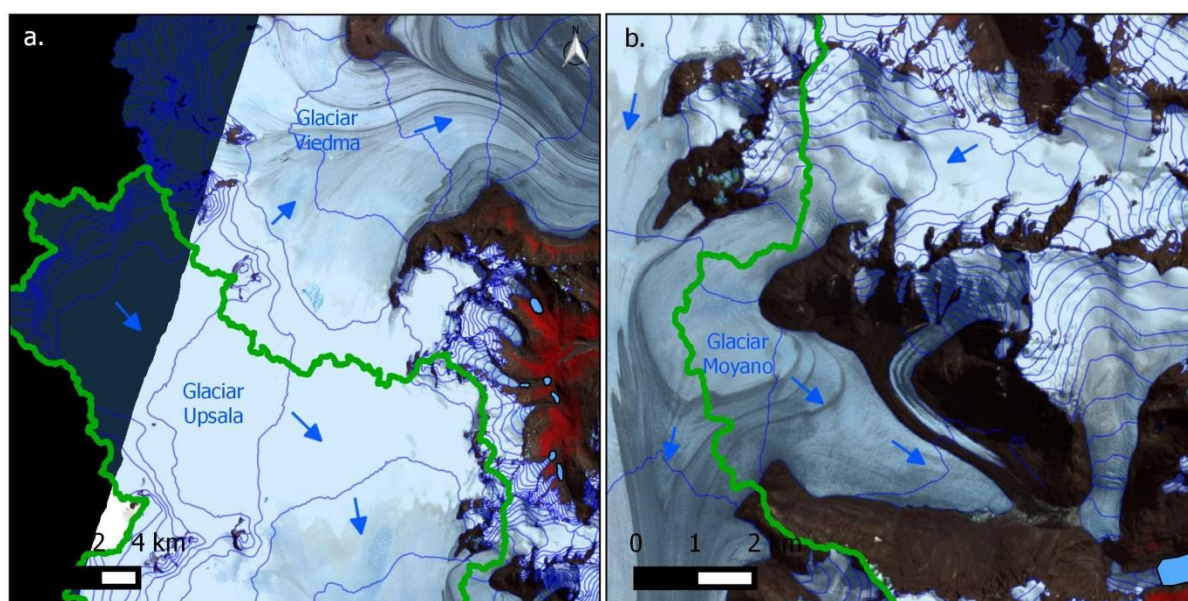
Figura 7: Divisoria de hielo. a: divisoria entre el glaciar Upsala y el glaciar Viedma. b: Glaciar Moyano con divergencia de flujo hacia dos cuencas. La forma sinuosa de la divisoria de hielo sobre los glaciares indica que la información topográfica no es precisa en esta zona.
