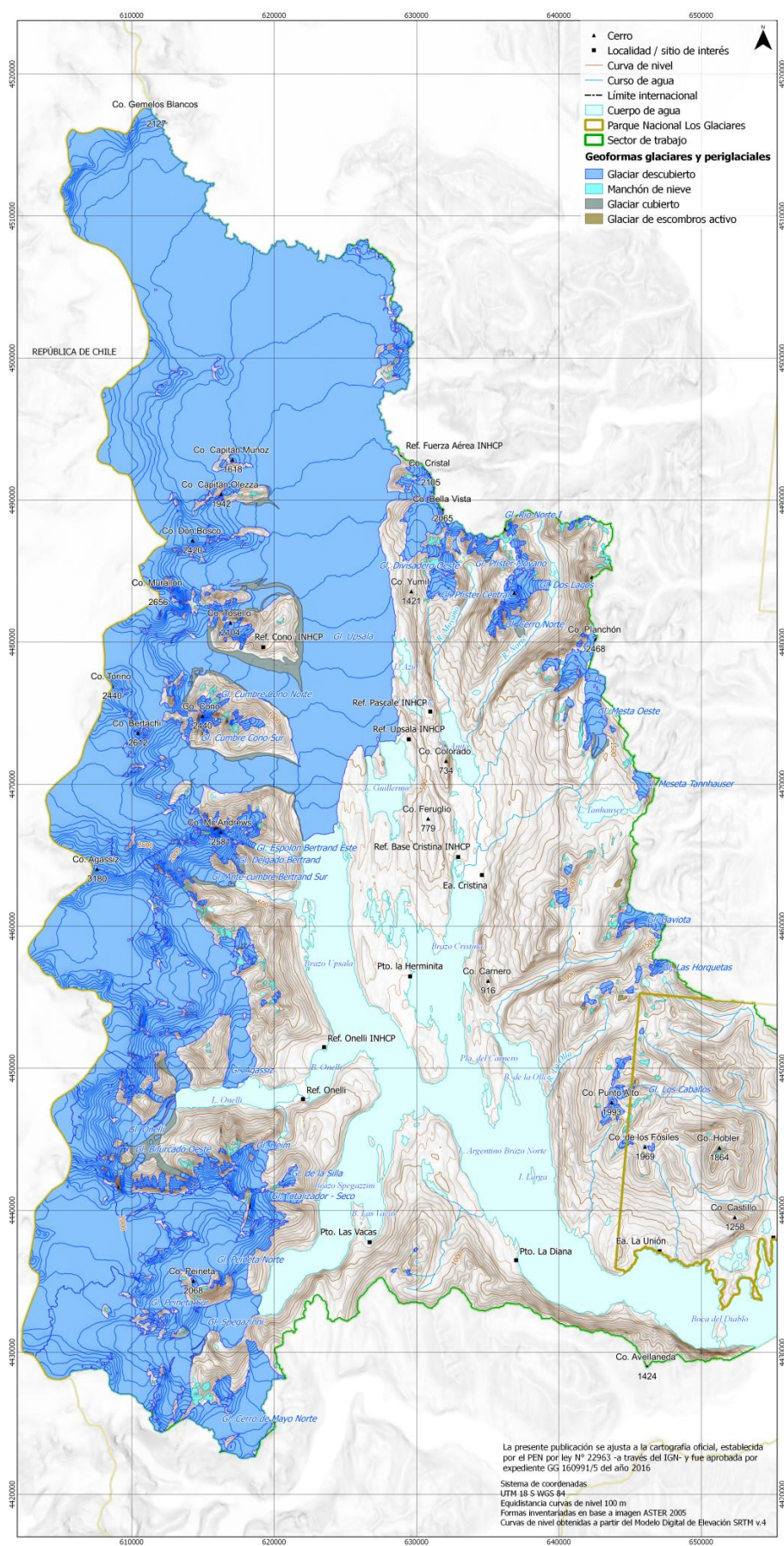
Figura 8: Mapa del inventario de glaciares.
