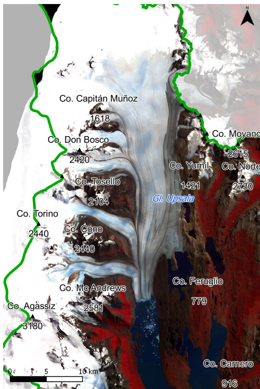
Figura 9: Glaciar Upsala y tributarios principales (imagen ASTER 20/02/2005).
