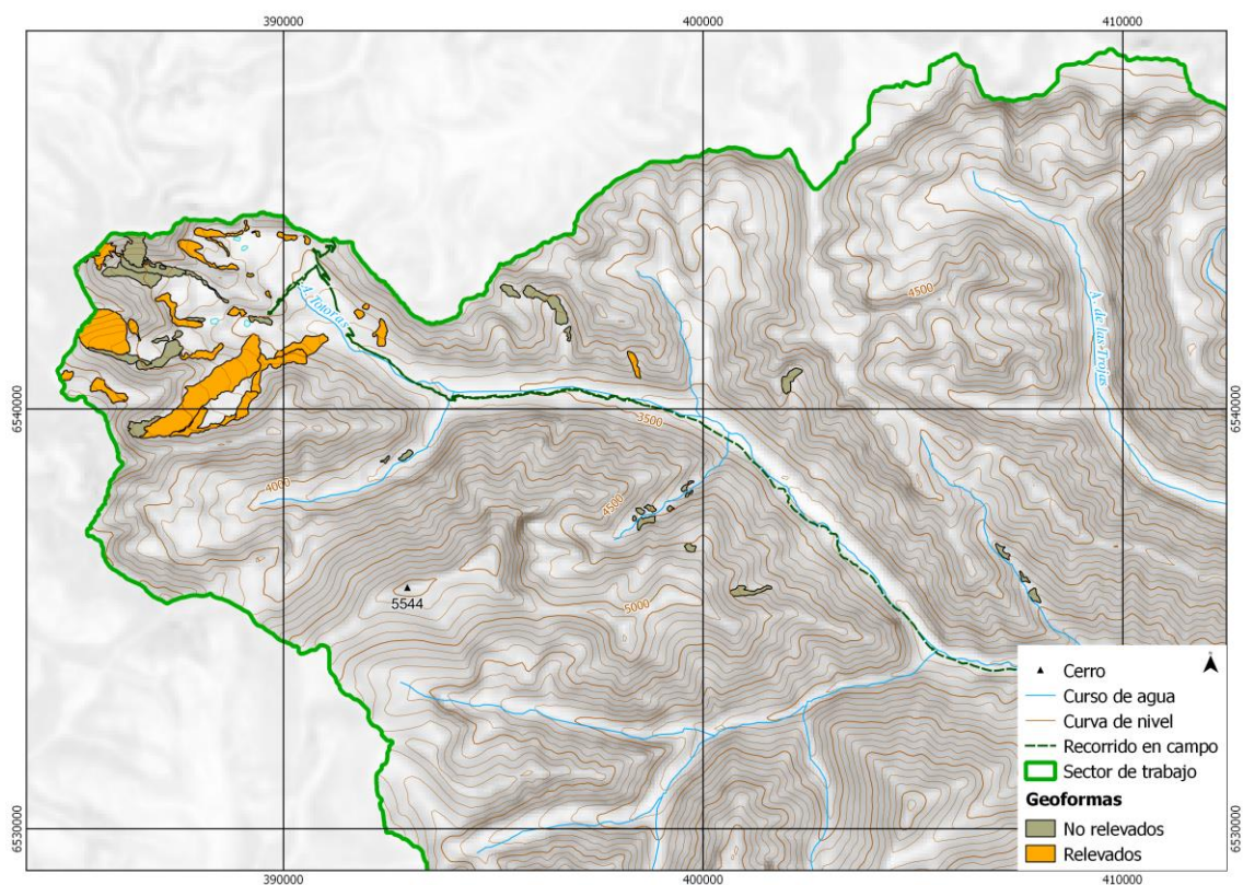
Glaciares relevados en el terreno. Sector de la subcuenca del río Calingasta.
