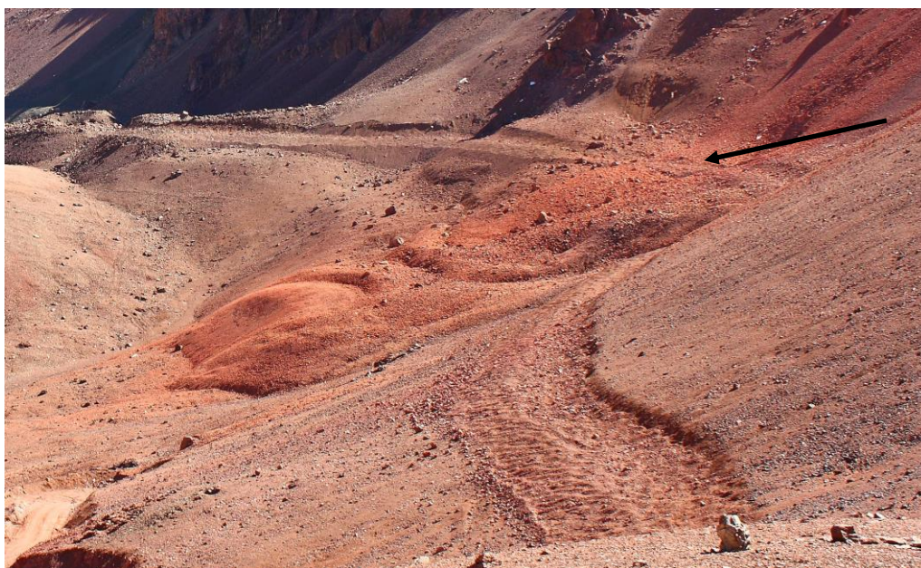
Detalle del frente de la geoforma (vista desde el sur)
