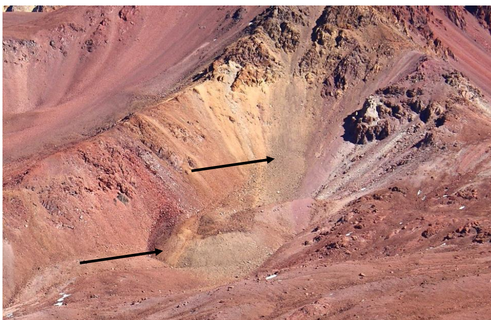
Detalles de la raíz y del talud de la geoforma G701634O312402S
