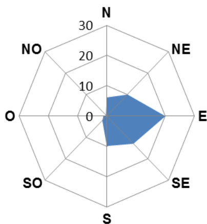
Figura 10: Orientación de los cuerpos de hielo inventariados en la subcuenca del río Calingasta.
