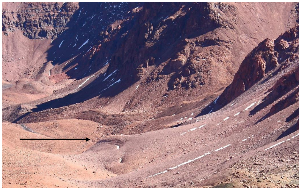
Detalle del talud de la geoforma G701616O312313S
