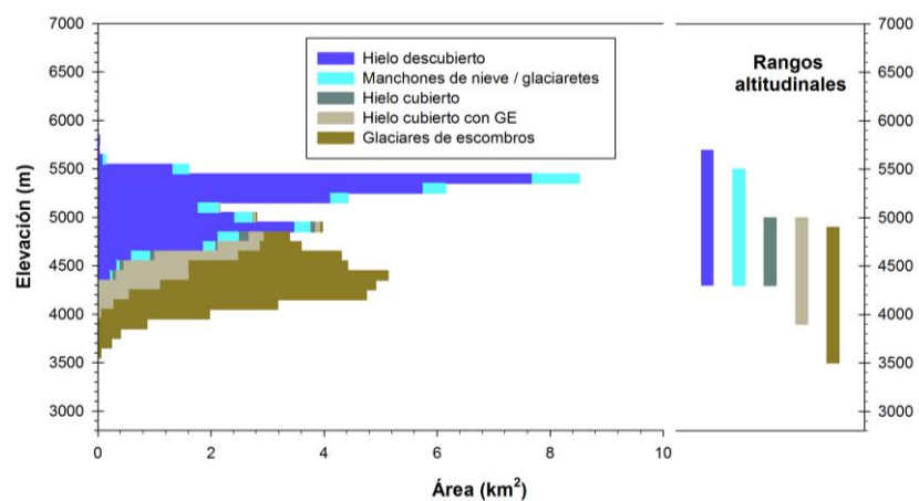
Figura 12: Hipsometría de los cuerpos de hielo, subcuenca del río Calingasta.
