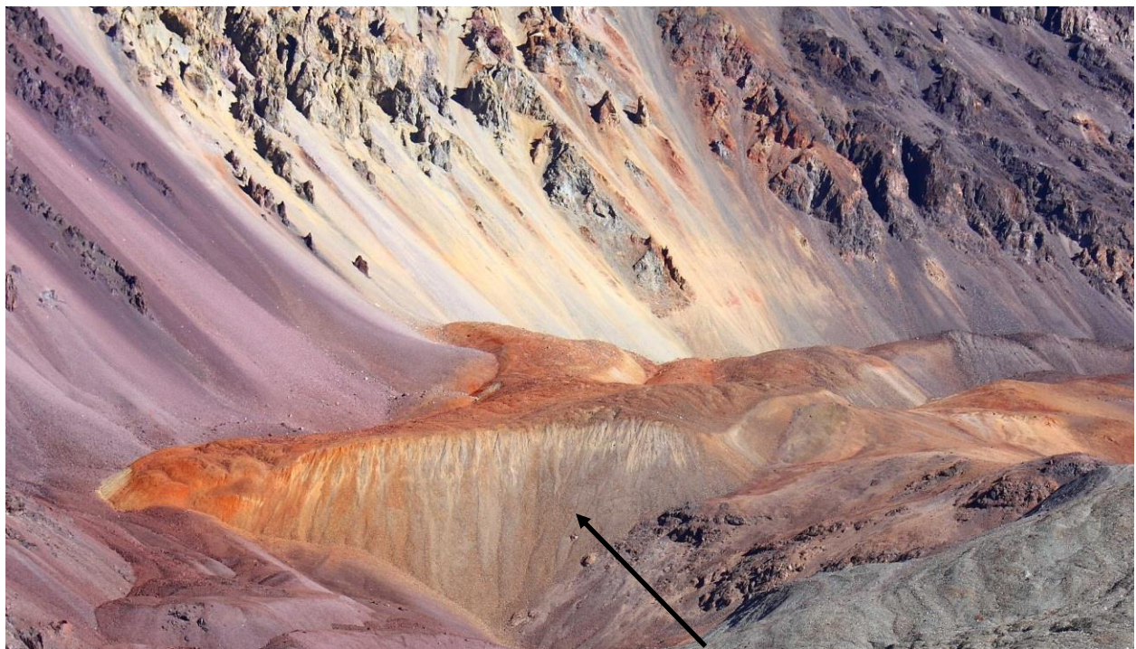
Detalle del talud de la Geoforma G701650O312681S
