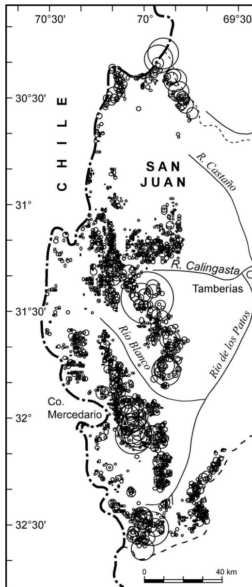
Figura 2: Inventario de glaciares de las cuencas de los ríos Castaño, Blanco y de los Patos, en la Provincia de San Juan, Bottero 2002.
