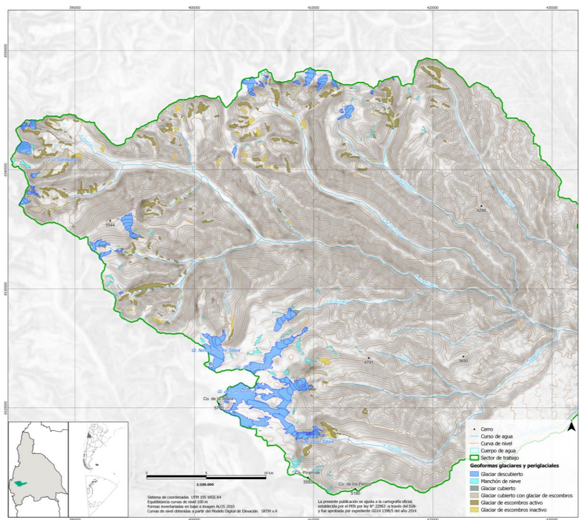
Figura 8: Glaciares en la subcuenca del río Calingasta.
