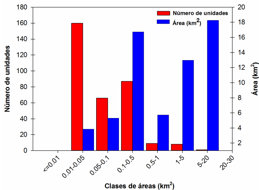
Figura 11: Distribución del número y superficie de los cuerpos de hielo, subcuenca del río Calingasta.
