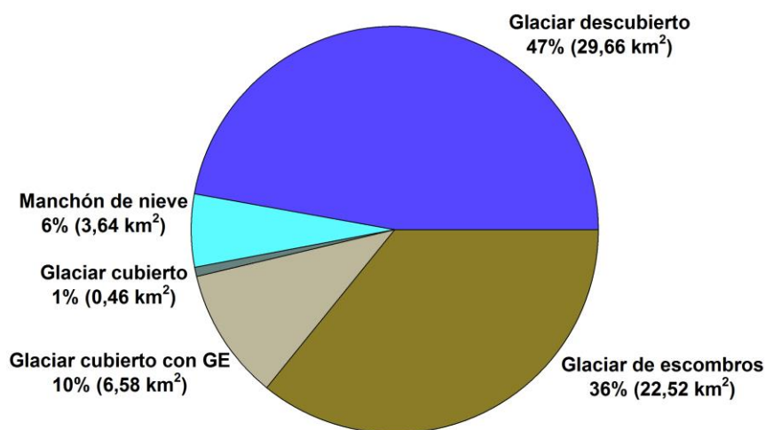
Figura 9: Distribución de los cuerpos de hielo inventariados, subcuenca del río Calingasta.
