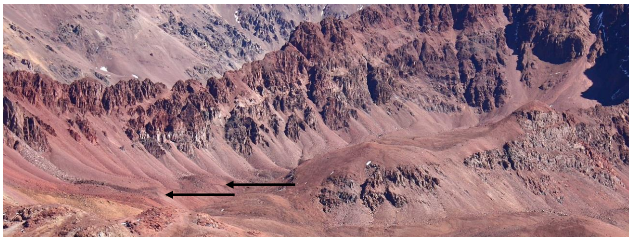
Detalle de los taludes de la geoforma G701775O312355S
