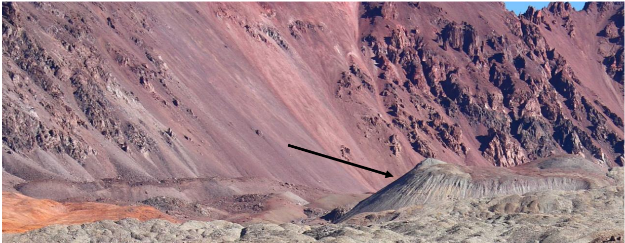
Detalle del talud de la geoforma
