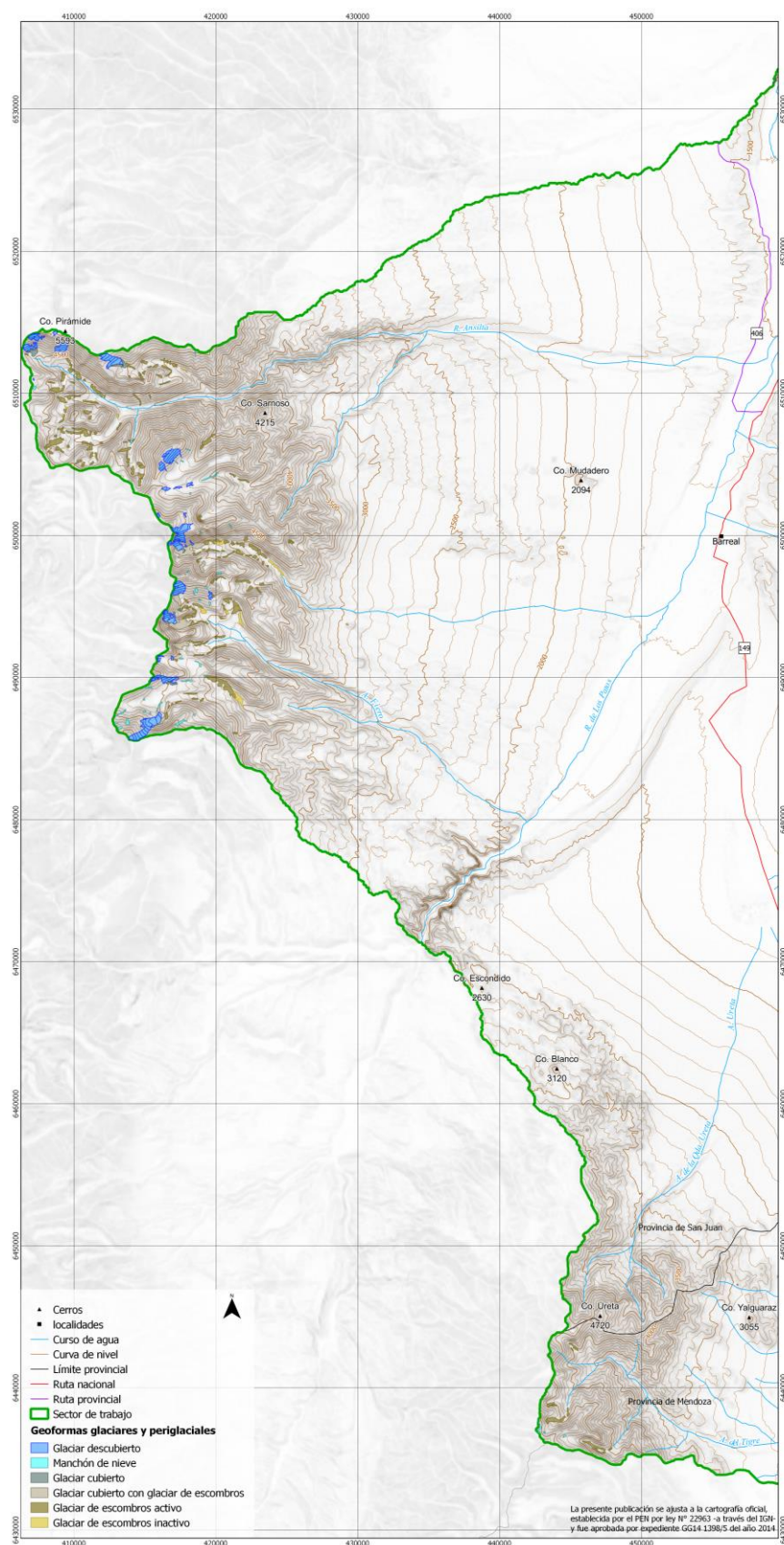
Figura 8: Glaciares en la subcuenca de la cordillera Ansilta.
