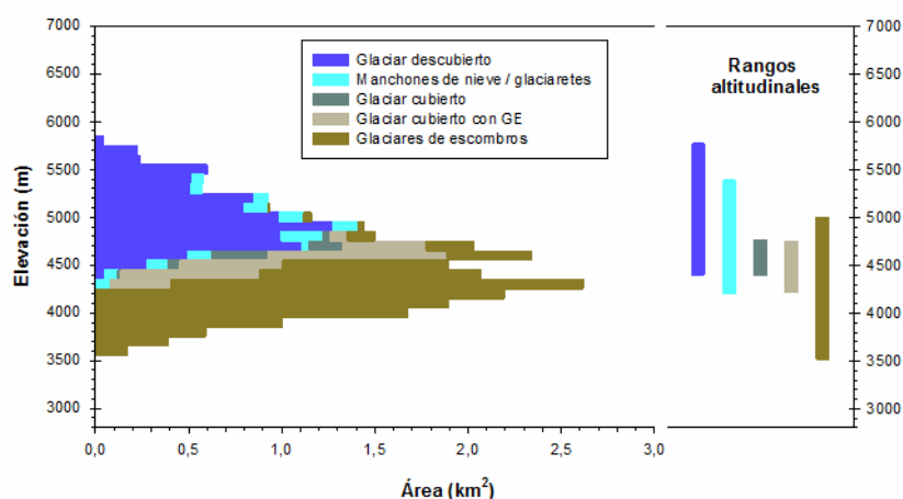
Figura 12: Hipsometría de los cuerpos de hielo, subcuenca de la cordillera Ansilta.
