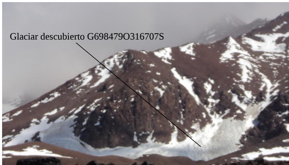
Pequeño glaciar de montaña G698479O316707S
