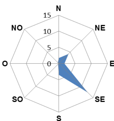
Figura 10: Orientación de los cuerpos de hielo inventariados en la subcuenca de la cordillera Ansilta.
