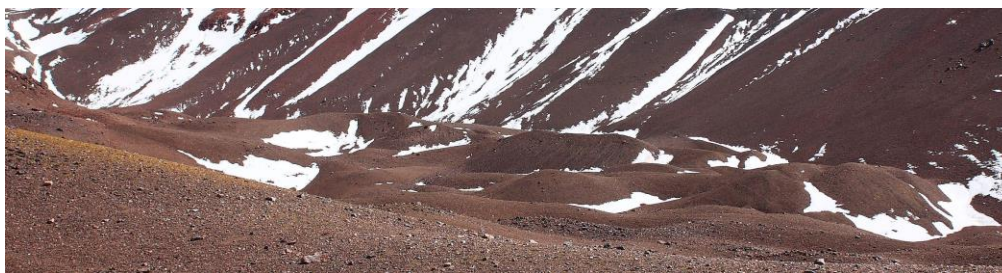
Glaciar de escombros inactivo G698551O316786S
