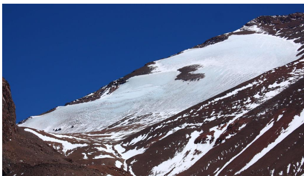
Glaciar descubierto G698551O316786S
