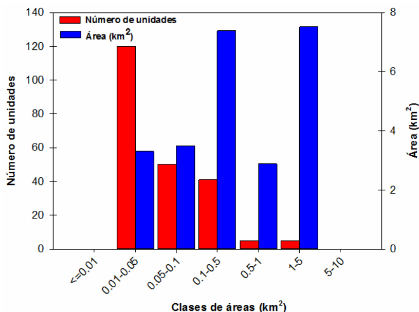
Figura 11: Distribución del número y superficie de los cuerpos de hielo inventariados, subcuenca de la cordillera Ansilta.
