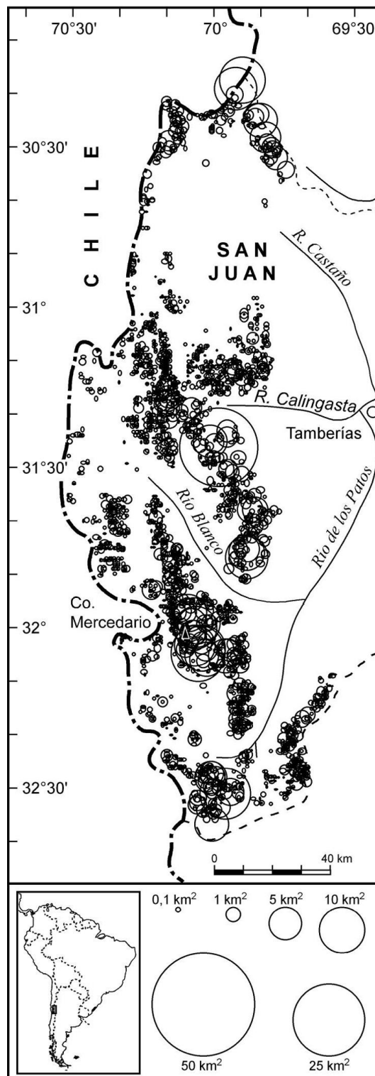
Figura 2: Inventario de glaciares de las cuencas de los ríos Castaño, Blanco y de los Patos, en la Provincia de San Juan, Bottero 2002.
