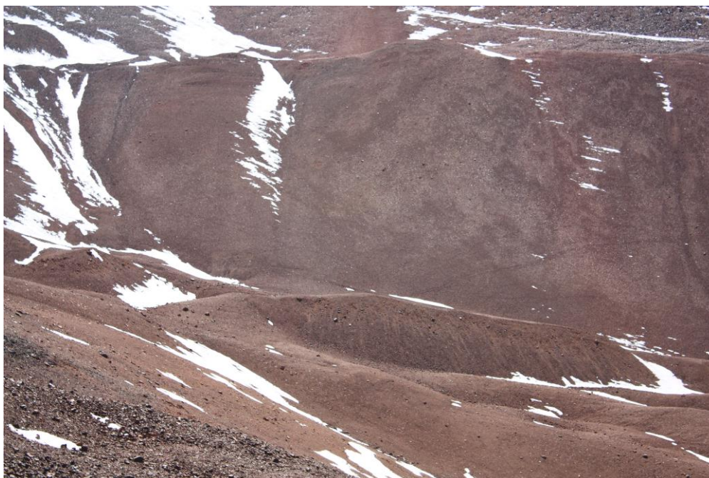
Glaciar de escombros activo G698551O316786S
