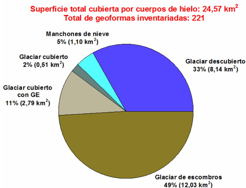
Figura 9: Distribución de los cuerpos de hielo inventariados, subcuenca de la cordillera Ansilta.
