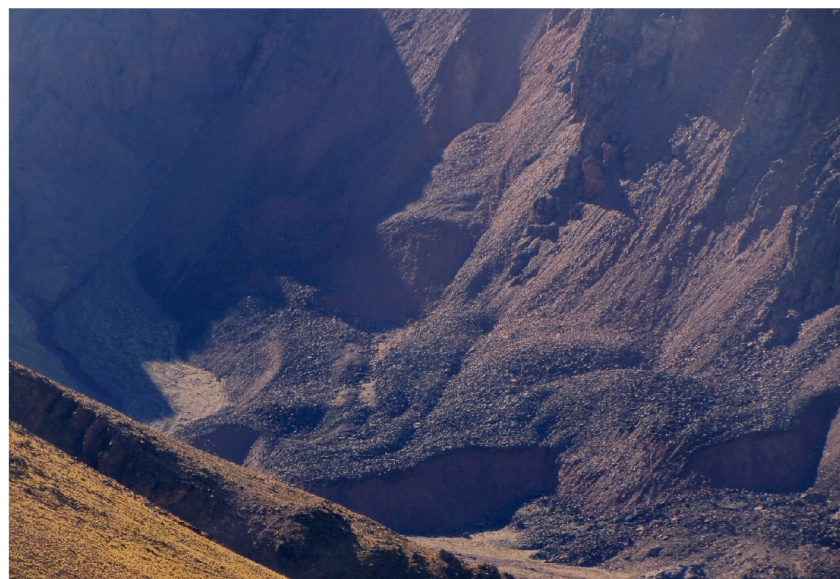
Glaciér de escombros en la Cordillera del Zenta (Foto: Lidia Ferri)
