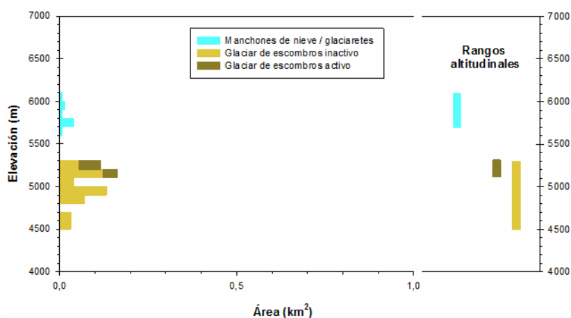
Figura 10: Hipsometría de los cuerpos de hielo, subcuenca Salar Pocitos.
