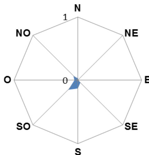
Figura 8: Orientación de los cuerpos de hielo inventariados en la subcuenca Salar Pocitos.
