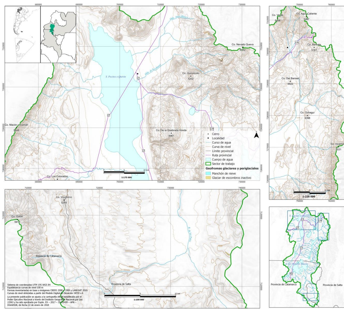
Figura 6: Cuerpos de hielo en la subcuenca Salar Pocitos.
