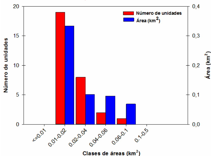
Figura 9: Distribución del número y superficie de los cuerpos de hielo inventariados por áreas en la subcuenca Salar Pocitos.
