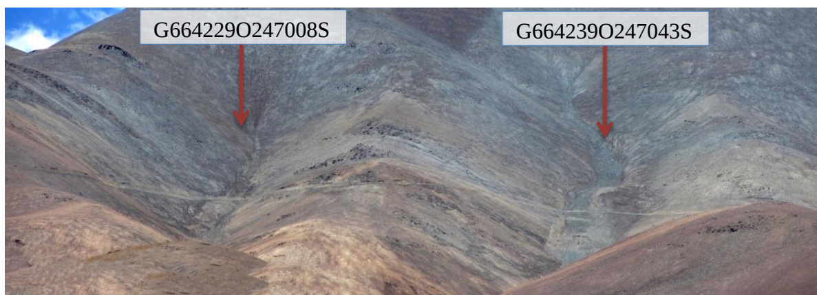
Glaciares de escombros inactivos G664229O247008S y G664239O247043S
