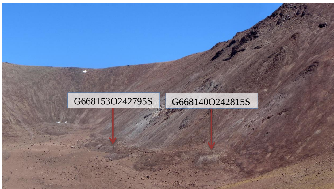
Detalle del frente del glaciar G668140O242815S
