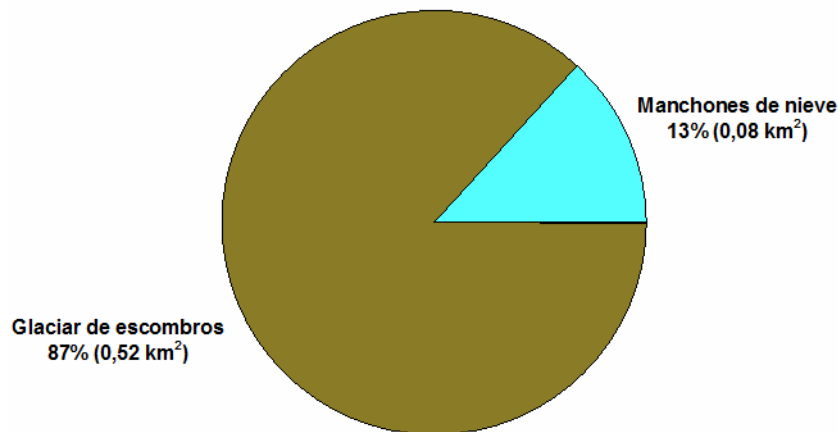
Figura 7: Distribución de los cuerpos de hielo inventariados, subcuenca Salar Pocitos.
