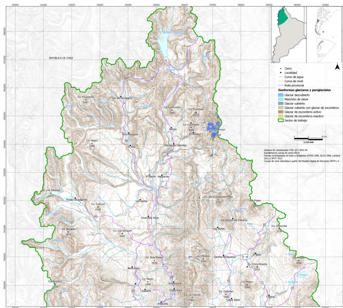
Figura 7: Inventario de glaciares de la subcuenca del río Neuquén norte.
