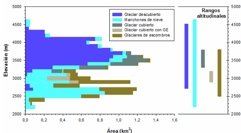
Figura 11: Distribución altitudinal (hipsometría) de los distintos cuerpos de hielo en la subcuenca del río Neuquén norte.
