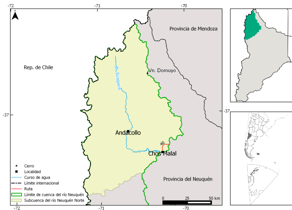
Figura 3: Subcuenca del río Neuquén norte, cuenca del río Neuquén, en la provincia homónima.
