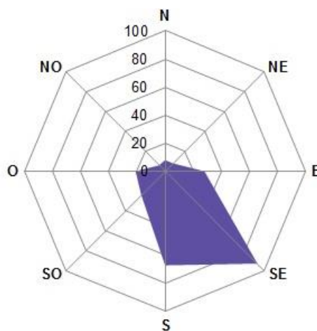
Figura 9: Orientación predominante de los cuerpos de hielo inventariados en la subcuenca del río Neuquén norte.
