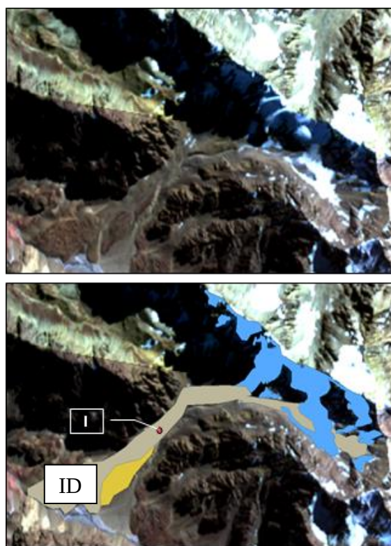
Figura 5: Ejemplo de una unidad compuesta vista en un mosaico de imágenes ASTER (arriba), y con todas las subunidades que la componen digitalizadas (abajo). El punto rojo en el centro de la unidad se utilizó para obtener las coordenadas geográficas de la misma. Todas las subunidades tienen el mismo código de identificación (ID).
