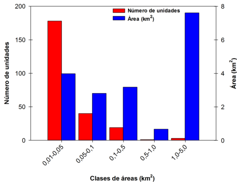
Figura 10: Distribución del número y superficie cubierta de los cuerpos de hielo inventariados en la subcuenca del río Neuquén norte, clasificada en categorías de acuerdo al tamaño de cada unidad.
