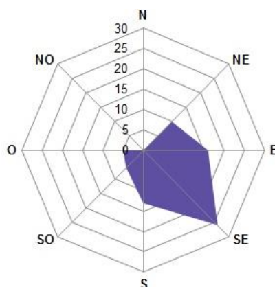
Figura 10: Orientación predominante de los cuerpos de hielo inventariados en las subcuencas de los ríos Collón Curá y Picún Leufú.
