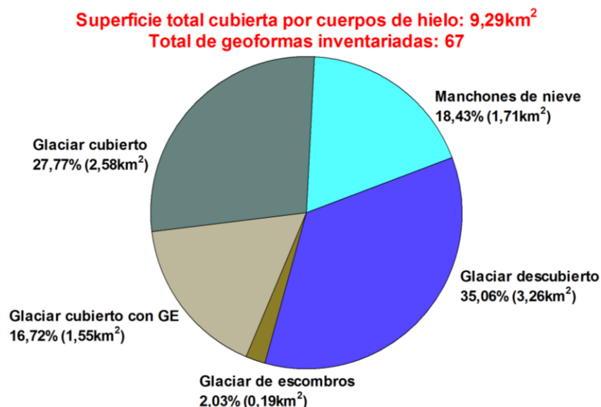
Figura 9: Tipos de cuerpos de hielo inventariados en las subcuencas de los ríos Collón Curá y Picún Leufú.
