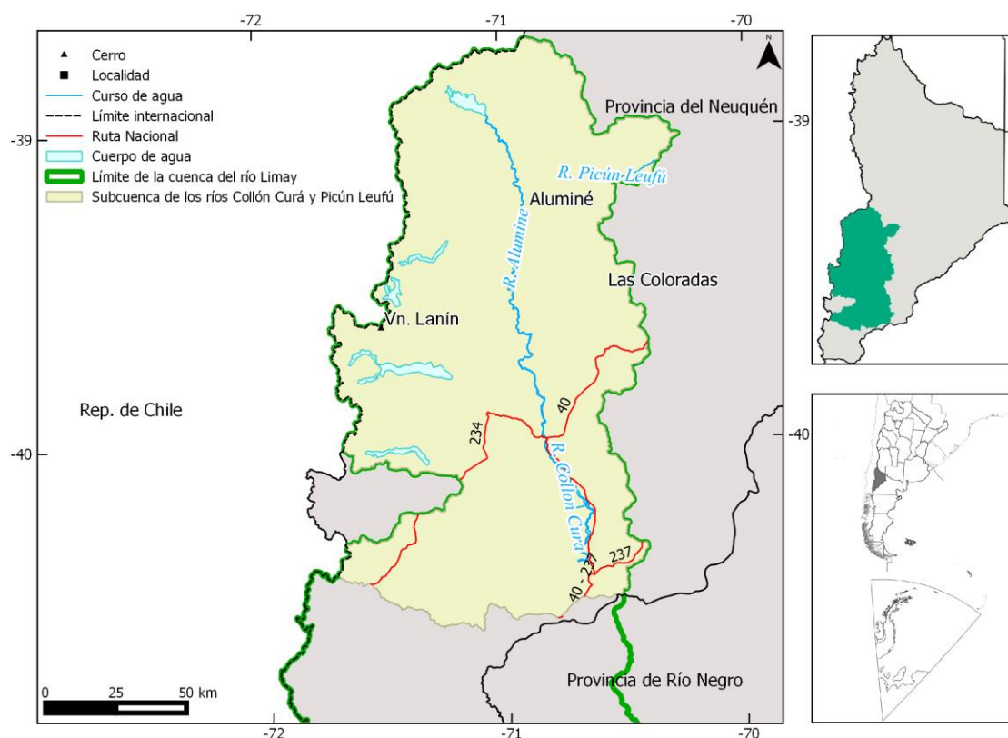
Figura 3: Subcuencas de los ríos Collón Curá y Picún Leufú, cuenca del río Limay, Neuquén.
