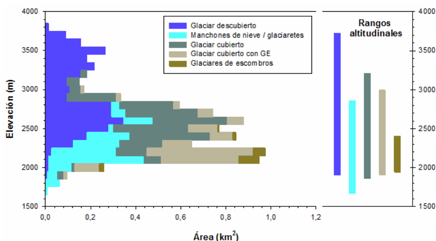
Figura 12: Distribución altitudinal (hipsometría) de los distintos cuerpos de hielo en las subcuencas de los ríos Collón Curá y Picún Leufú.
