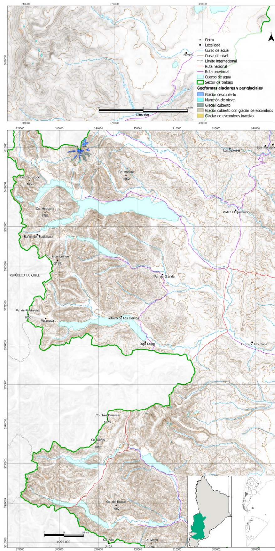
Figura 8: Inventario de glaciares de las subcuencas de los ríos Collón Curá y Picún Leufú.
