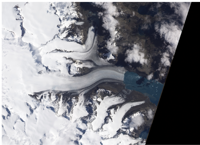
Glaciar Neumayer captado por el satélite ALI, NASA's Earth Observing-1
