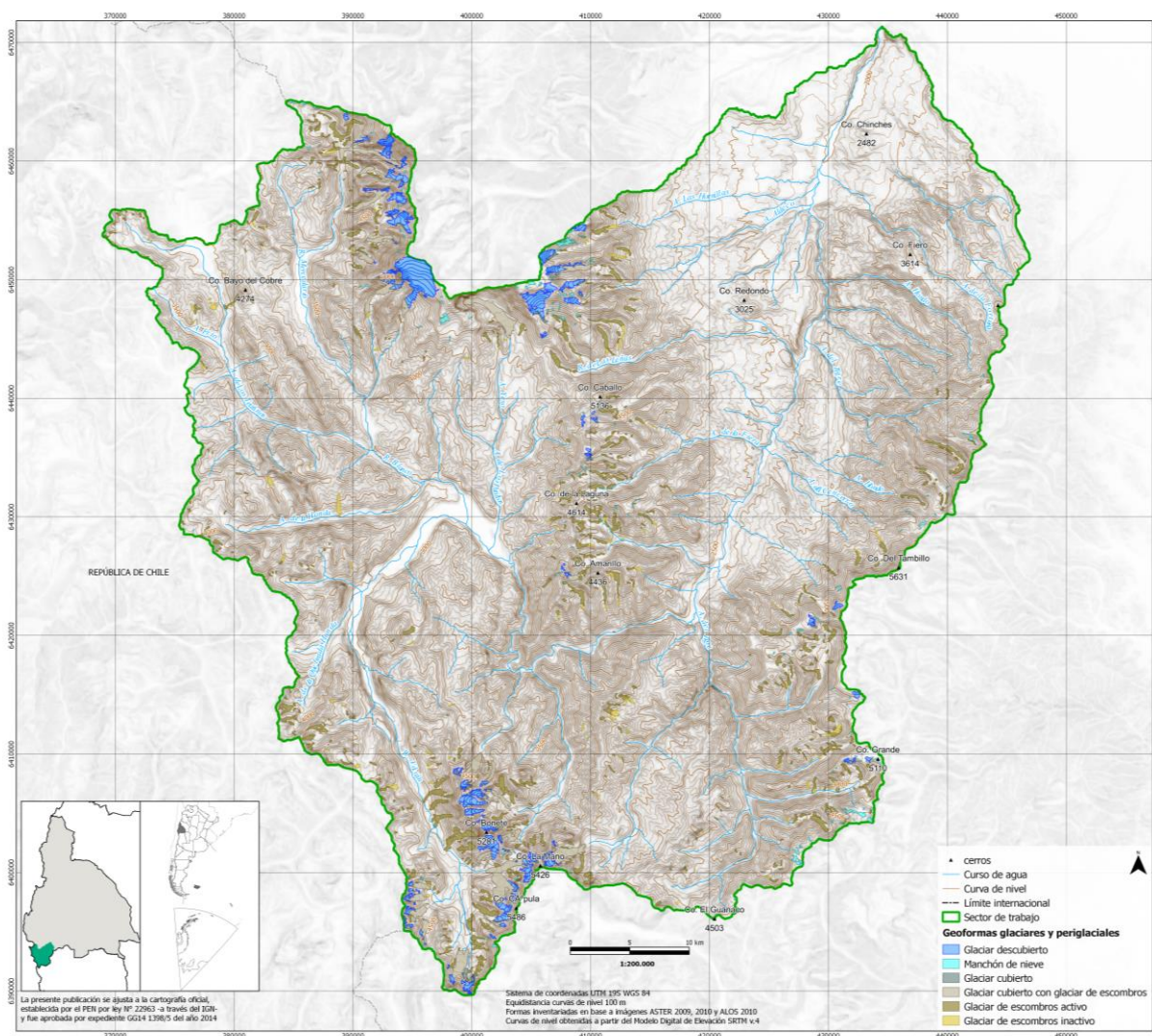
Figura 9: Glaciares en la subcuenca del río de Los Patos.
