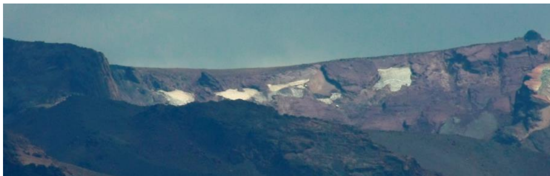
Manchón de nieve G705423O371881S
