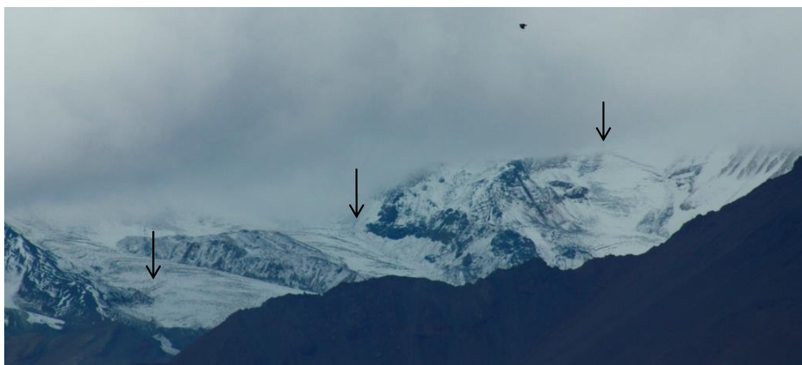
Glaciar descubierto G704678O366255S
