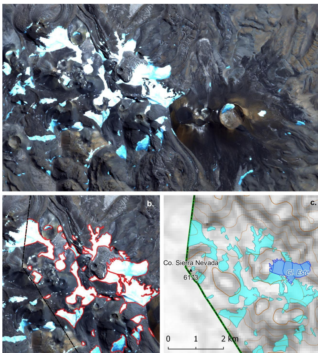
Figura 4: Delimitación en forma manual del hielo descubierto en el área del Co. Sierra Nevada. Imagen ALOS-AVNIR 2: Glaciar Este (G685505O264930S) y manchones de nieve alrededor del cerro. b) Cuerpos de hielo digitalizados manualmente. c) Mapa final del inventario.
