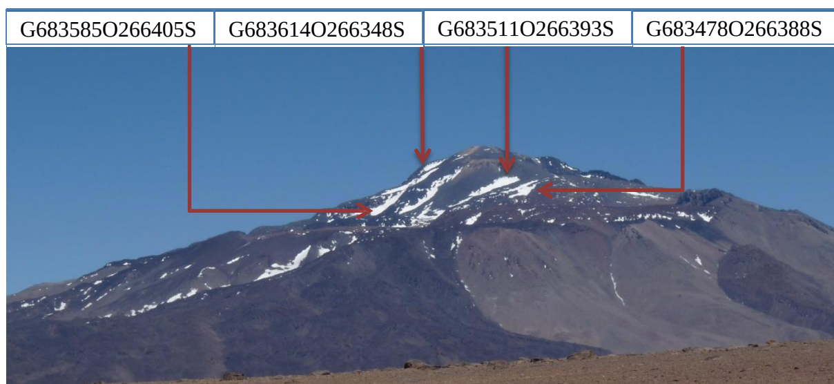
Panorámica de los manchones de nieve ubicados sobre ladera sur de cerro El Cóndor.
