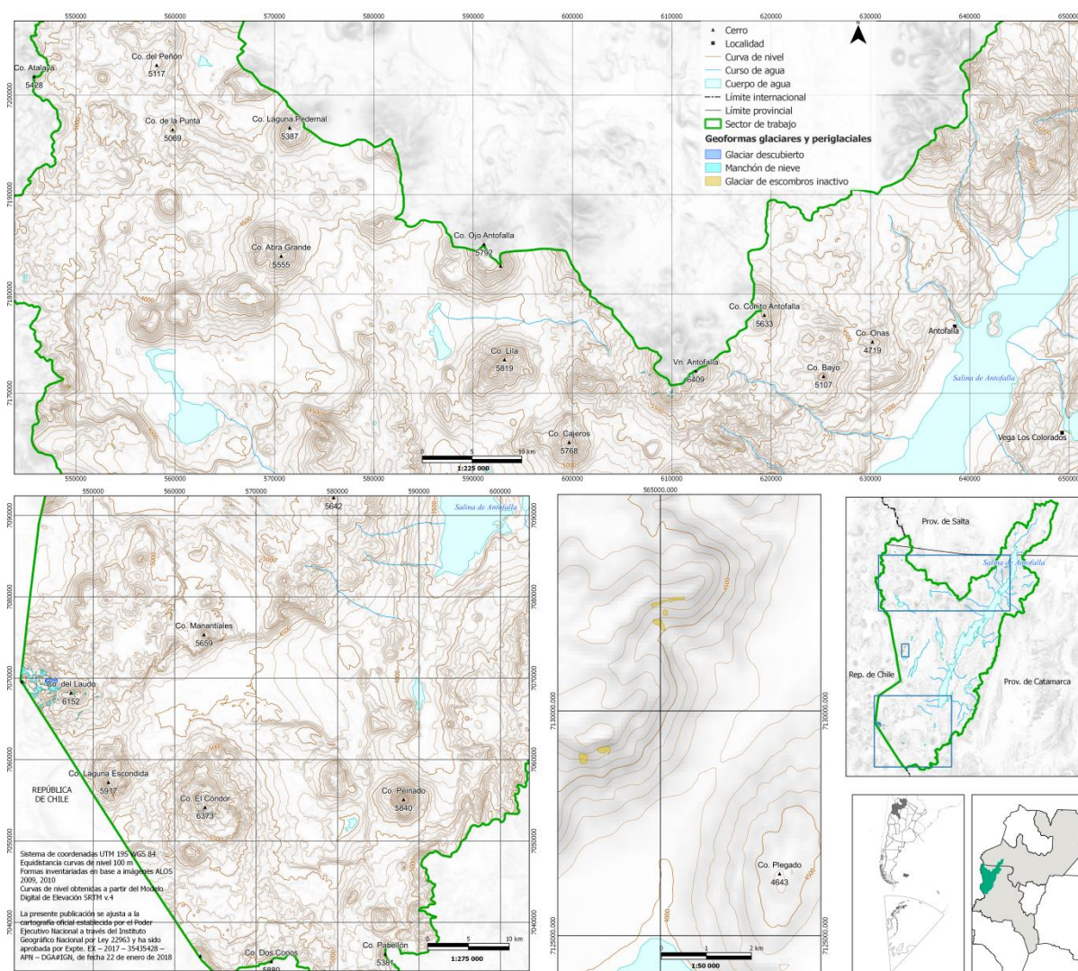
Figura 6: Cuerpos de hielo en la subcuenca Salar de Antofalla.
