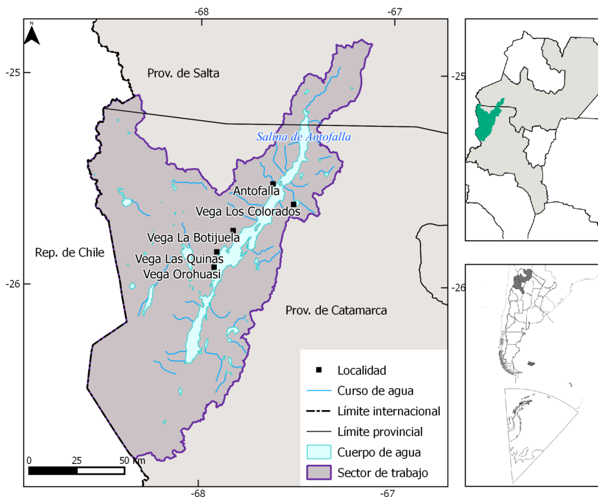
Figura 2: Mapa de ubicación de la subcuenca Salar de Antofalla.
