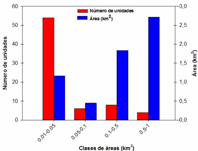
Figura 9: Número de unidades y superficie cubierta por los cuerpos de hielo inventariados en la subcuenca Salar de Antofalla.
