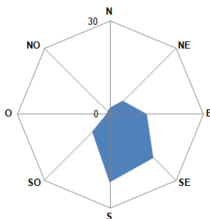
Figura 8: Orientación de los cuerpos de hielo inventariados en la subcuenca Salar de Antofalla.
