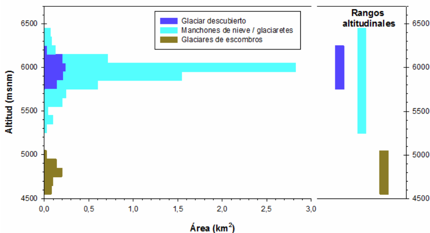
Figura 10: Hipsometría de los cuerpos de hielo, subcuenca Salar de Antofalla.
