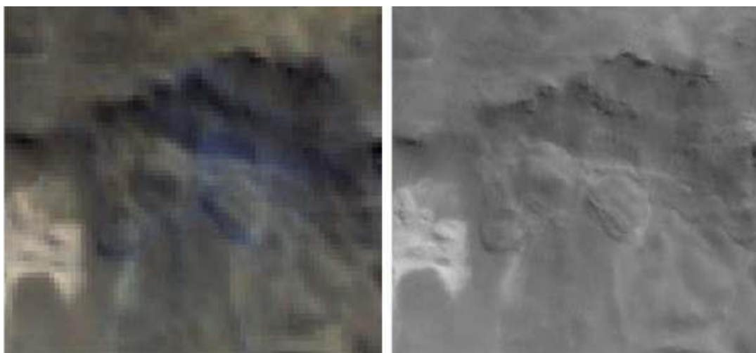
Figura 5: Ejemplo de la importancia de la resolución espacial de las imágenes en la identificación de crioformas. En la parte izquierda puede observarse un glaciar de escombros (G669843O263928S) en una imagen SPOT5 (10 m de resolución). A la derecha se puede apreciar la misma crioforma con mayor detalle en una imagen CBERS2 de 2,5 m de resolución espacial.
