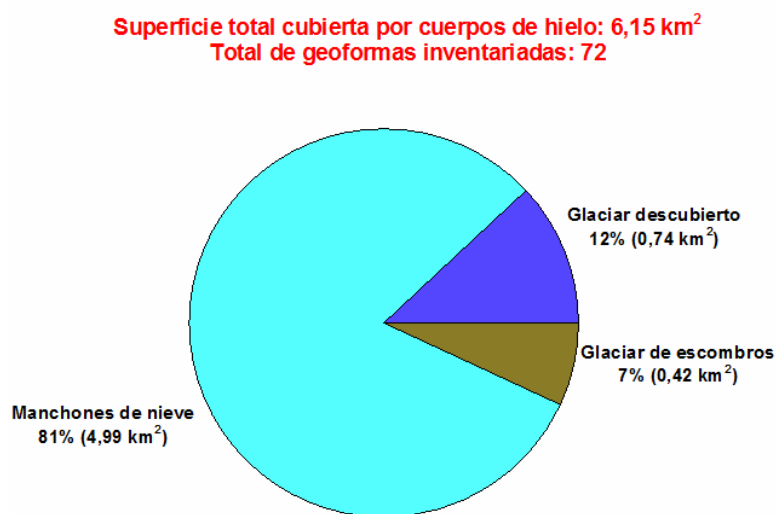
Figura 7: Distribución de los cuerpos de hielo inventariados, subcuenca Salar de Antofalla.
